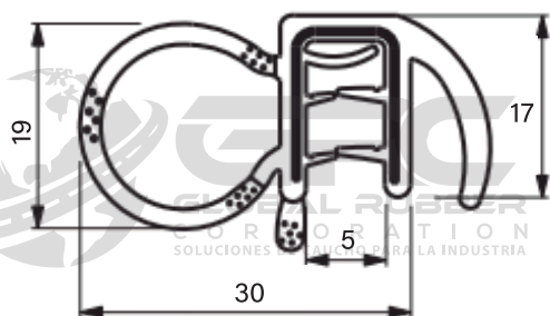
Perfil Burlete Alambrado 150
