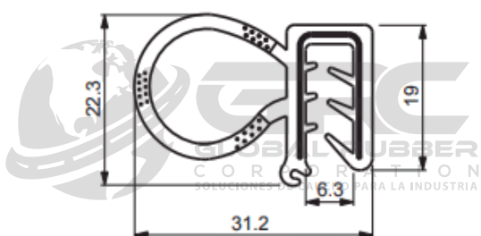
Perfil Burlete Alambrado 384
