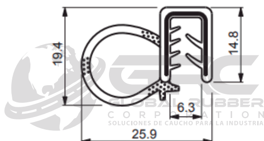
Perfil Burlete Alambrado 373
