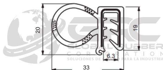
Perfil Burlete Alambrado 375
