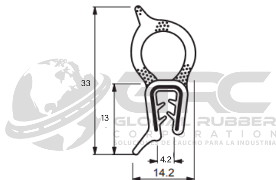
Perfil Burlete Alambrado 341
