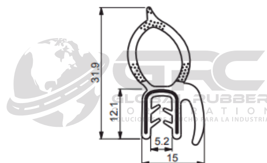
Perfil Burlete Alambrado 374
